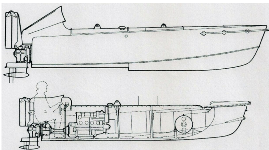
Рис. 1. Схема итальянского катера камикадзе MT (сверху) и его модифицированной версии МТМ (внизу) (Italian МТМ)
