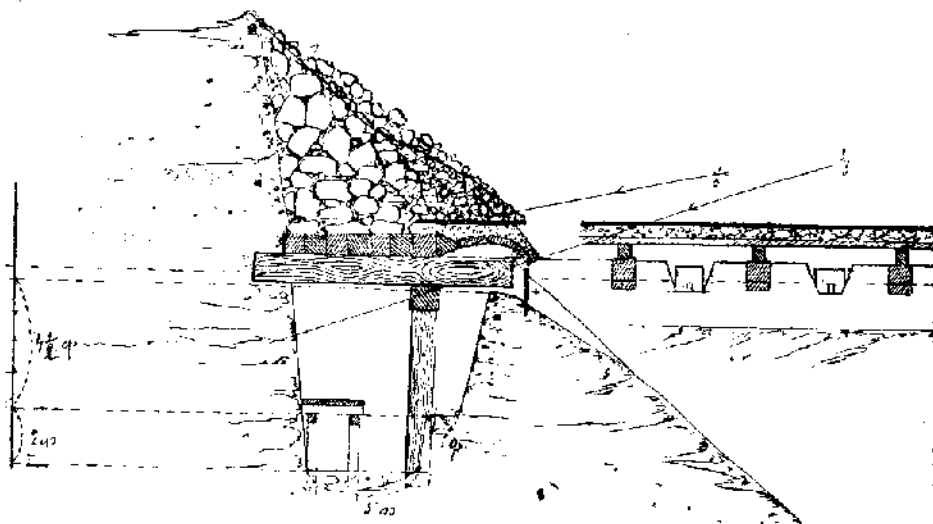
Профиль для самыхъ крутыхъ отлогостей при скалистомъ грунтѣ.
