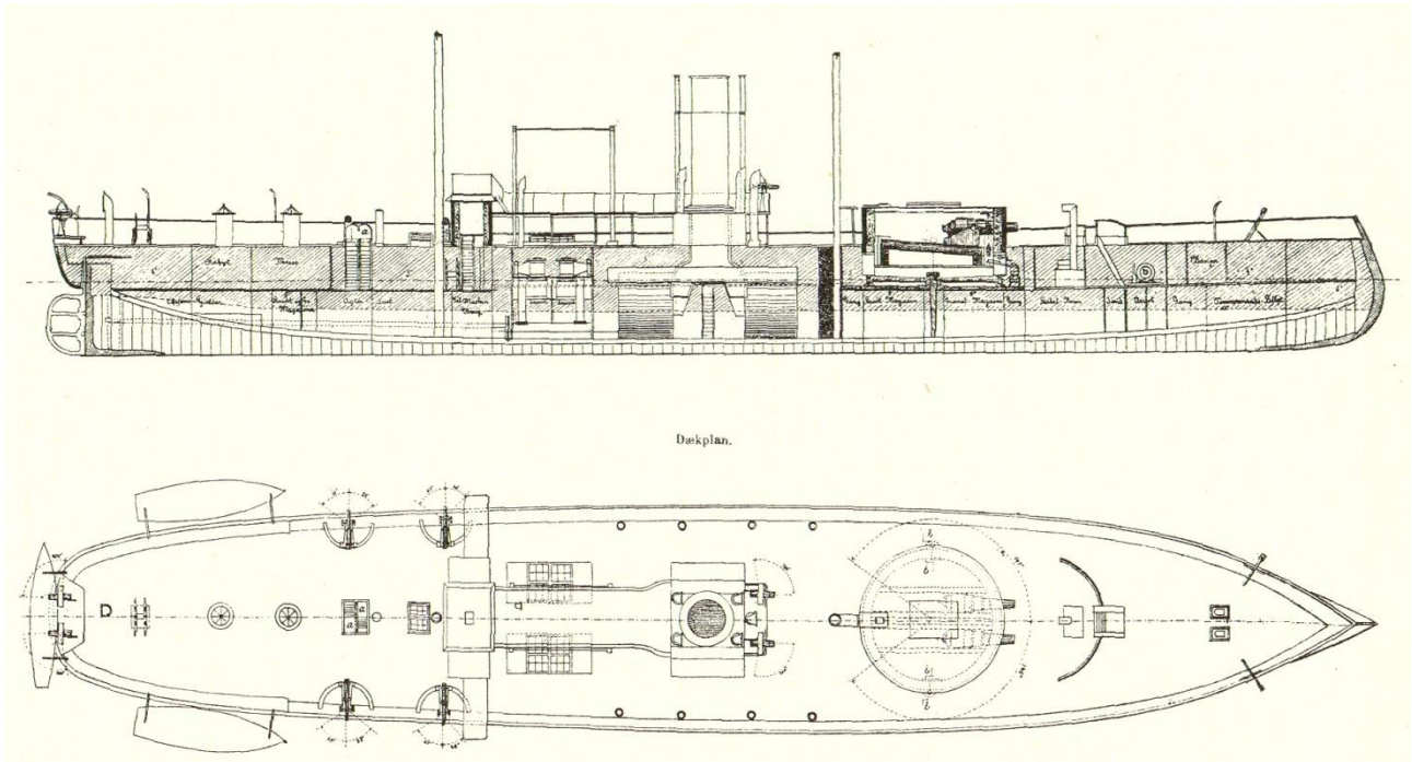
Схема монитора "Линдормен"
