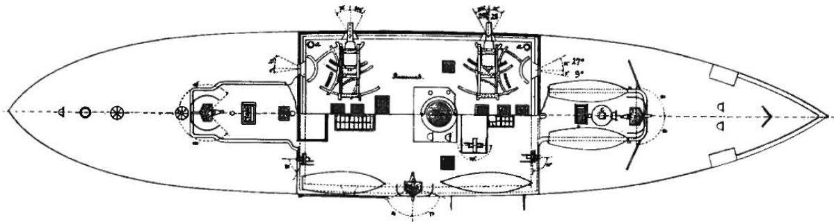
Первоначальная схема броненосца "Один"
