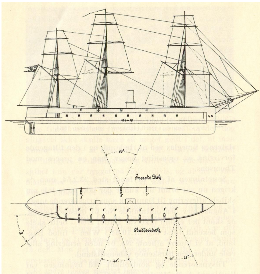
Схема броненосца "Данмарк"
